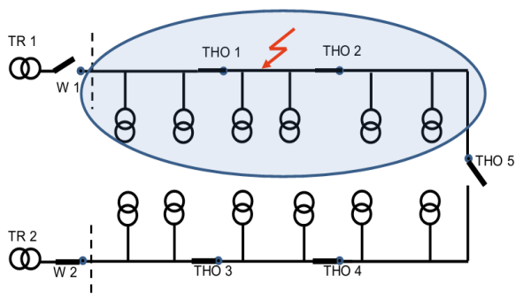
Rys. 3. Model linii SN wyposażonej w rozłączniki THO z uszkodzeniem na linii gdzie: THO1...THO5 – rozłączniki radiowo w głębi sieci SN
