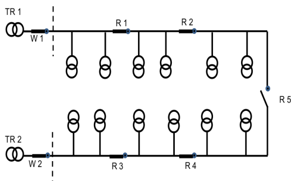
Rys. 1. Model linii SN w układzie normalnym gdzie: W1 i W2 – wyłączniki w GPZ-cie, R1...R5 –reklozery w głębi sieci SN
