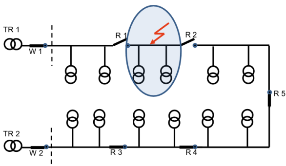
Rys. 2. Model linii SN z wyeliminowanym miejscem uszkodzenia
